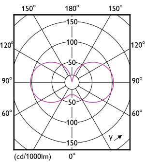
Light Distribution Diagram - 5B11/PER/CRI95WG/FR/G/E12/WGD 1CT T20
