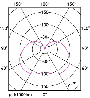
Light Distribution Diagram - LEDStick 6W E27 DS FR ND 1CT/6 AU
