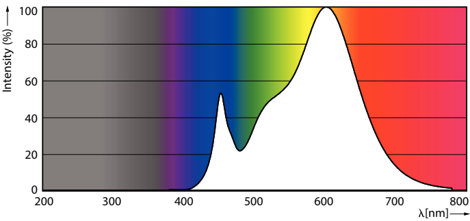
Spectral Power Distribution Colour - LEDStick 6W E27 DS FR ND 1CT/6 AU
