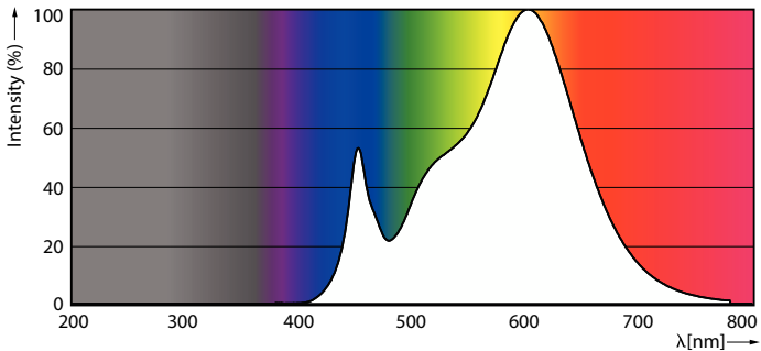
Spectral Power Distribution Colour - LEDStick 6W B22 DS FR ND 1CT/6 AU
