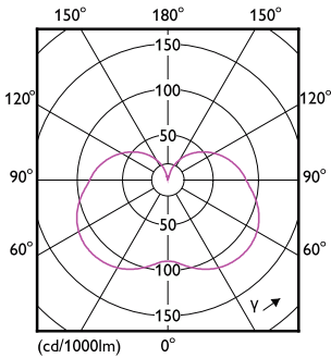
Light Distribution Diagram - LEDStick 6W B22 DS FR ND 1CT/6 AU
