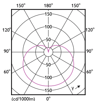
Light Distribution Diagram - LEDBulb 8W E27 DS FR ND 1CT/6 AU
