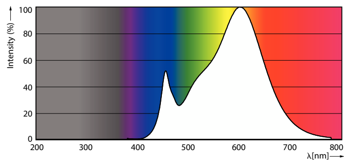
Spectral Power Distribution Colour - LEDBulb 8W E27 DS FR ND 1CT/6 AU
