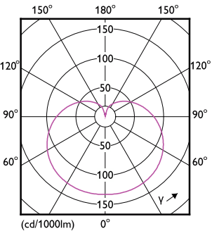
Light Distribution Diagram - LEDBulb 8W B22 DS FR ND 1CT/6 AU
